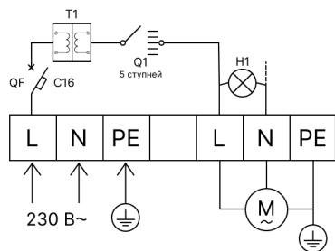
Схема подключения
