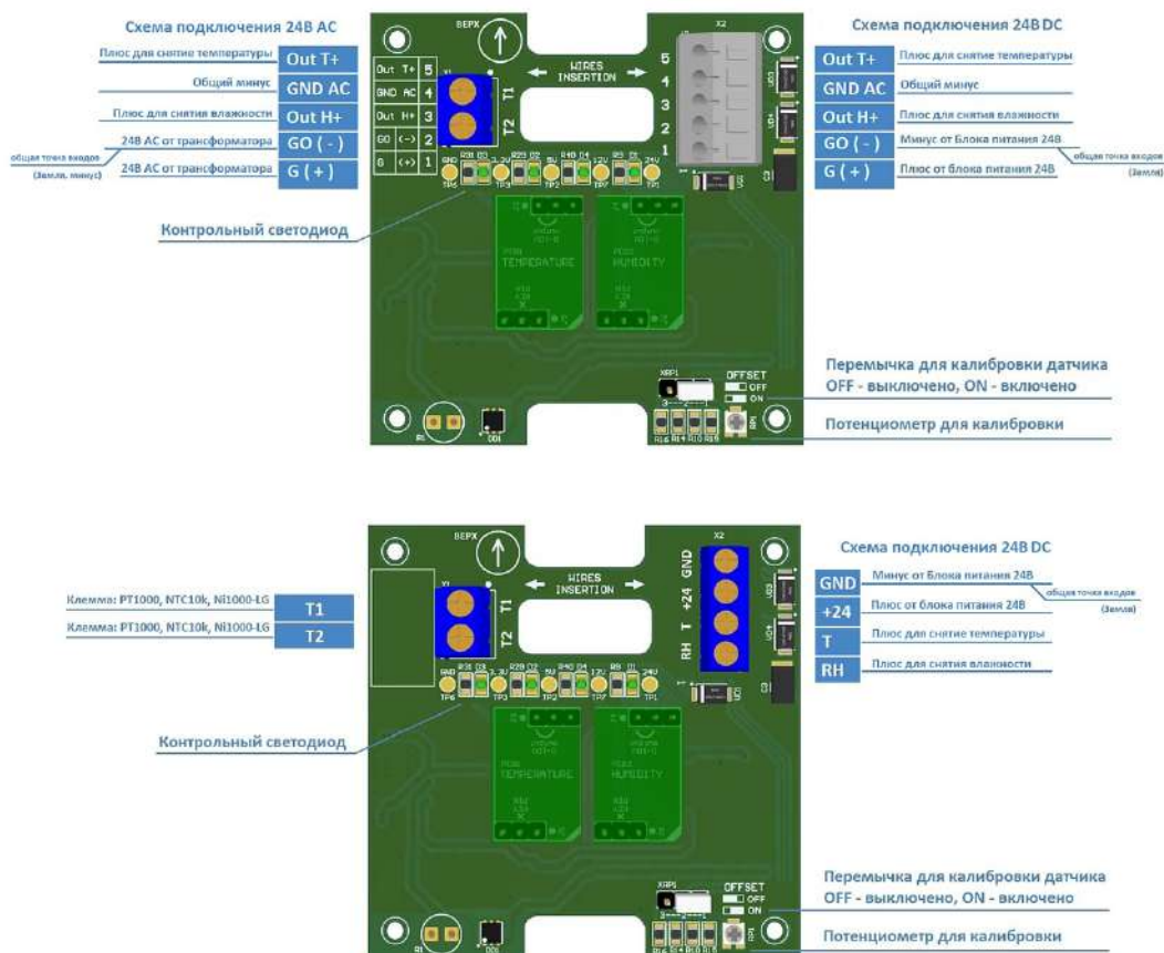
Табл. 3 Подключение датчика влажности (верхний рисунок для датчиков 24 В AC/DC, нижний только 24 В DC)
